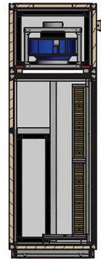
A-A ( 1 :30 )
